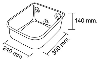
COMEDERO ACERO INOXIDABLE, 6 litros
